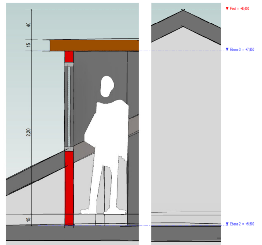
Schnitt A
