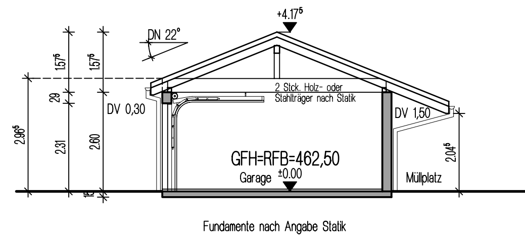
Schnitt B-B Garage
